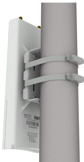
Рисунок 10 — Крепление устройства к трубостойке
