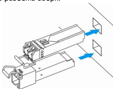
Рисунок 66 – Установка SFP-трансиверов
